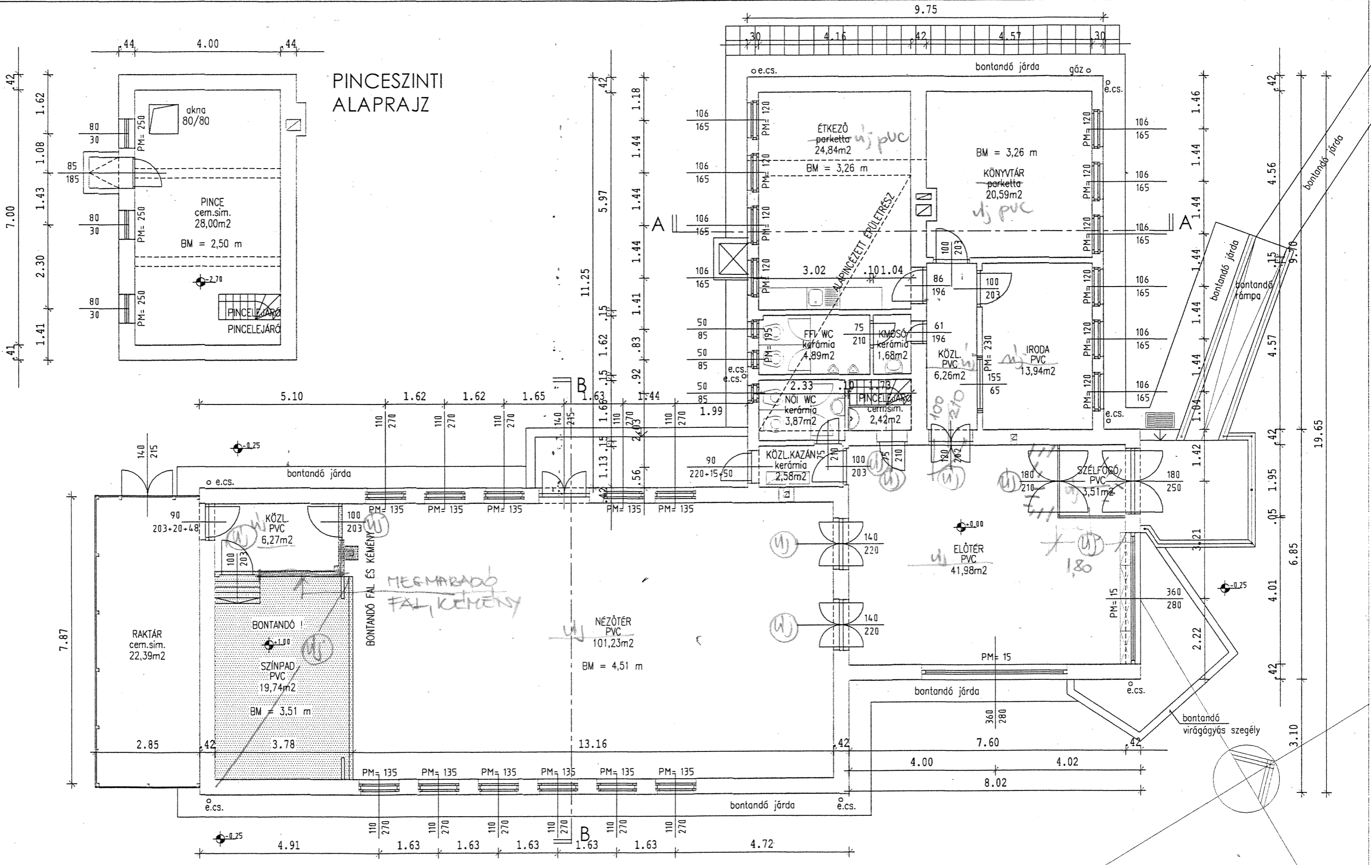
FÖDSZINTI ALAPRAJZ
